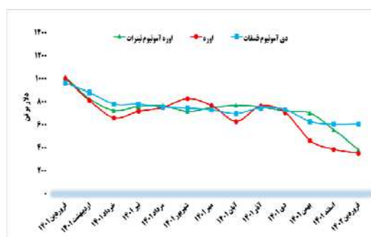
نمودار (۳): روند تغییرات ماهانه قیمت جهانی انواع کود شیمیایی در بورس کالای جهانی مأخذ: tradingeconomics.com
